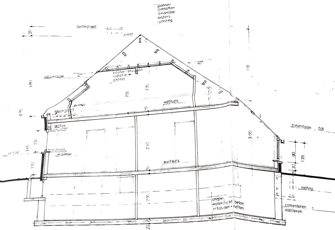
DOORSNEDE A.B.
