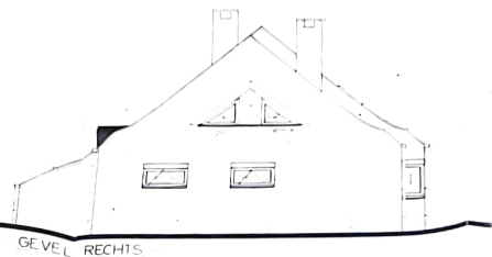
GEVEEL RECHTIS
