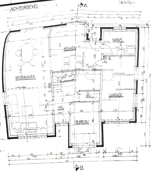
PLAN GELIJKVLOERS
